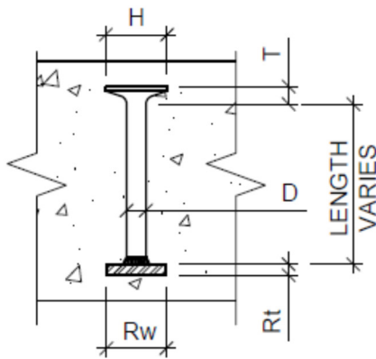
SECTION 1-1 N.T.S
